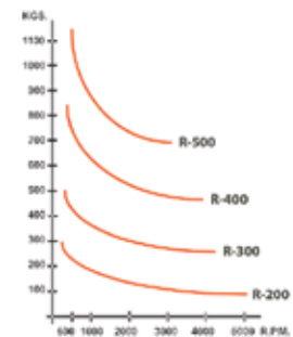
CARGA AXIAL 2.000 horas de vida
