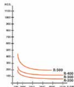
CARGA AXIAL 2.000 horas de vida
