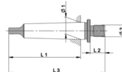
Espigas roscadas UNF
